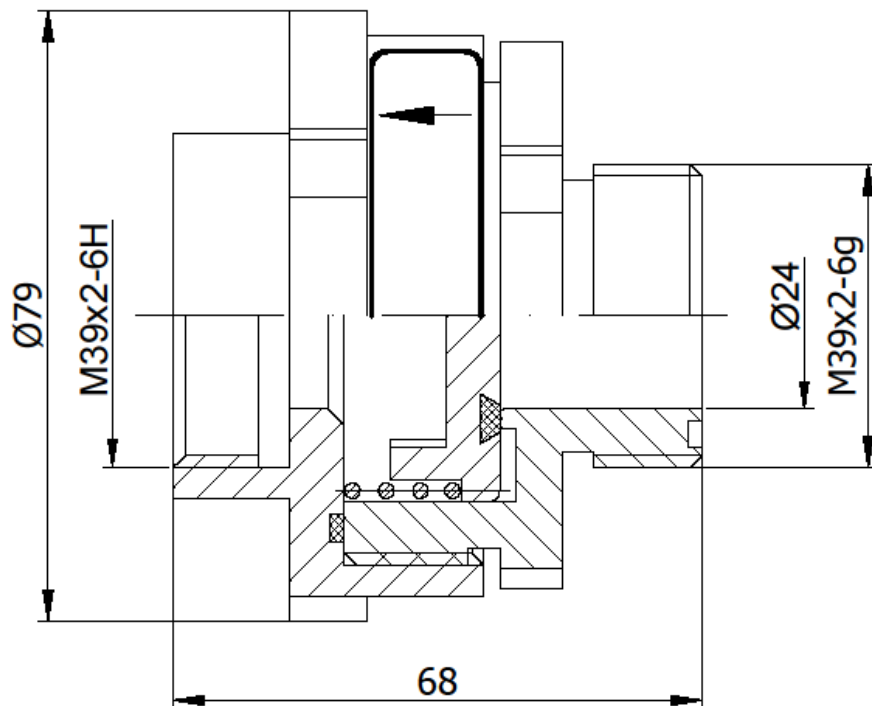
Рисунок 1 – Общий вид клапана обратного коллектора КО-24-150
