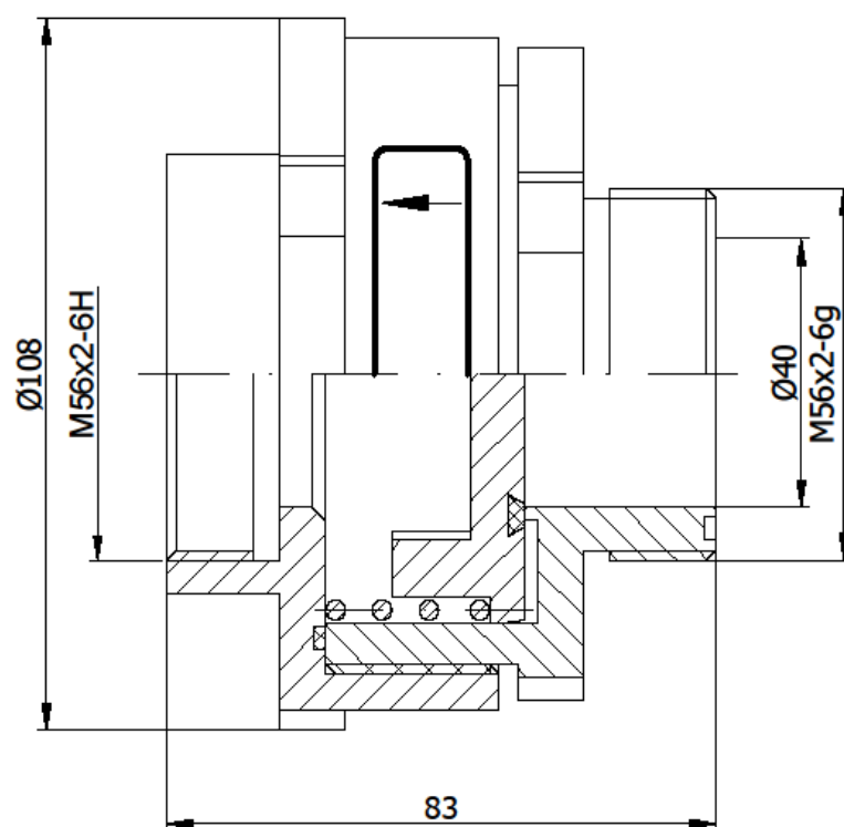
Рисунок 1– Общий вид клапана обратного коллектора КО-40-150
