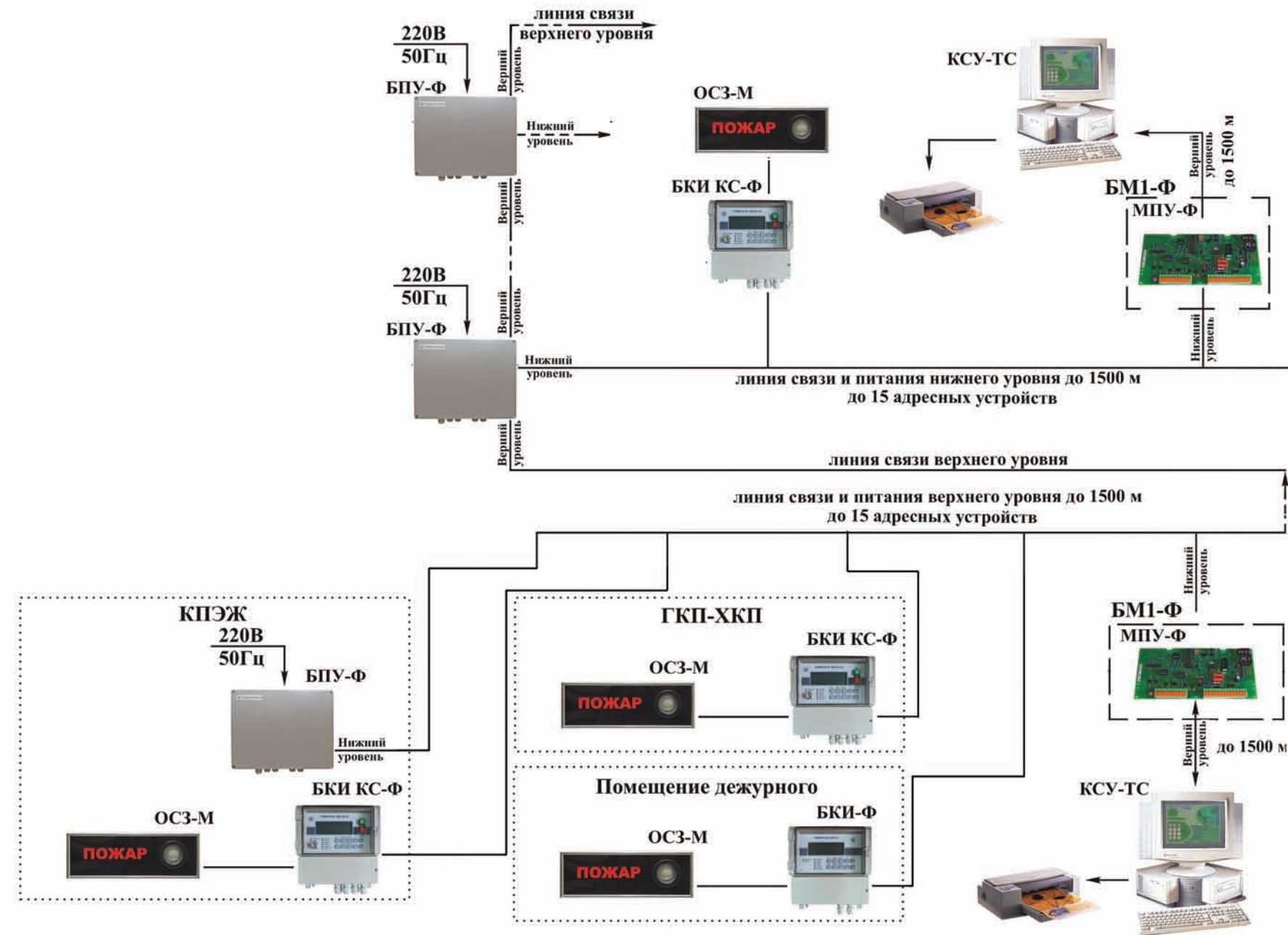
Структурно-функциональная схема объёмного химического тушения
