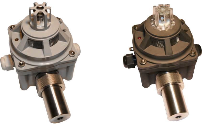
Рис. 44 ИП 212/101/435-«Барк М-Г» («Галион»). Общий вид
