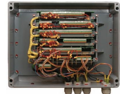
Рис. 27 БМ5-Ф. Общий вид со снятой крышкой
