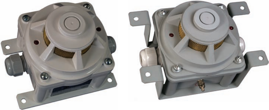
Рис. 31 ИП212-«Фрегат М». Общий вид с пластинами
