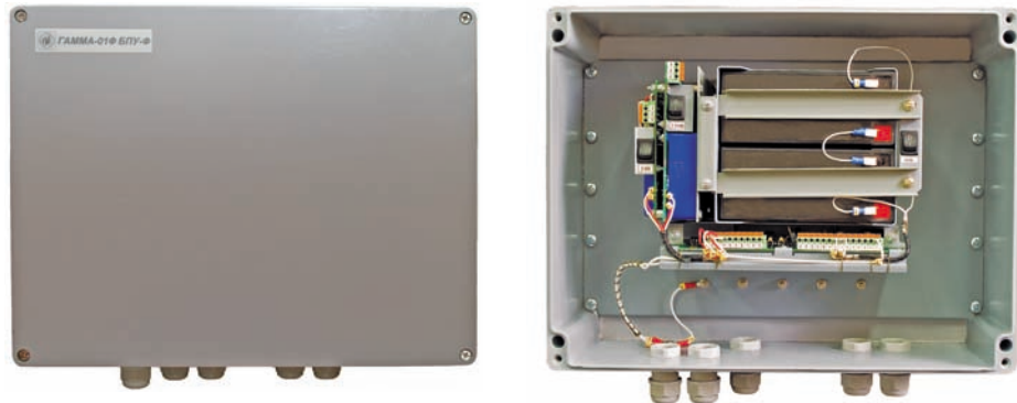
Рис. 1 БПУ-Ф. Общий вид Рис. 2 БПУ-Ф. Общий вид со снятой крышкой
