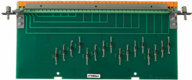
Рис. 22 МР. Общий вид
