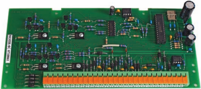
Рис. 17 МОПИ-Ф. Общий вид
