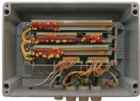
Рис. 25 БМ3-Ф. Общий вид со снятой крышкой
