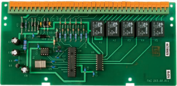
Рис. 18 МРВ. Общий вид
