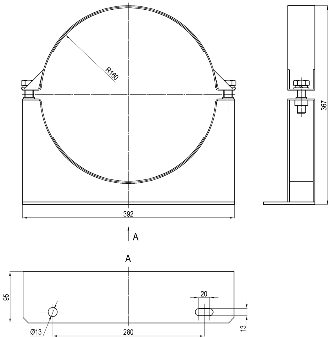
Рисунок 1 – Общий вид хомута сейсмостойкого
