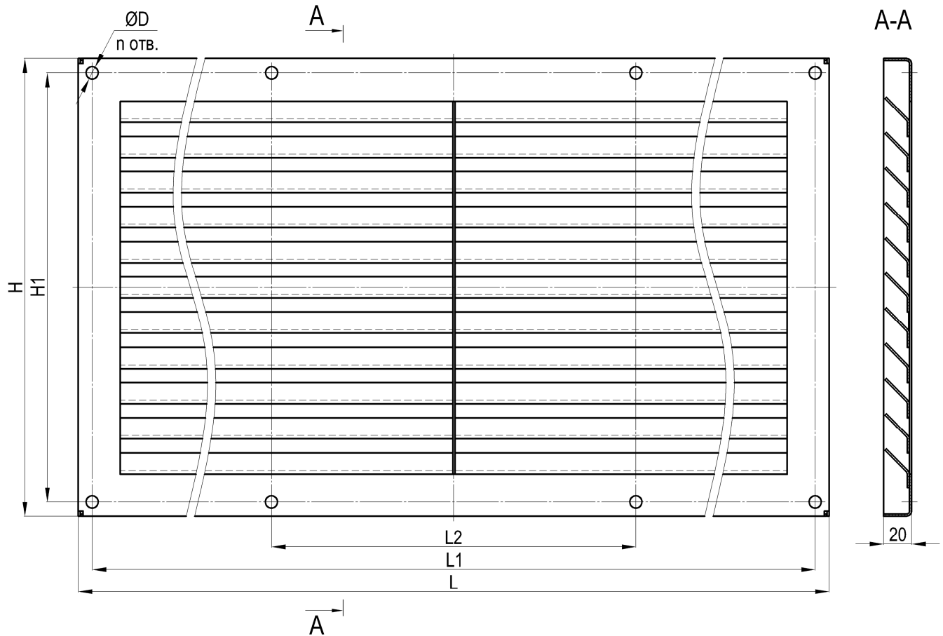
Рисунок 1 – Общий вид решетки Р-КСИДв
