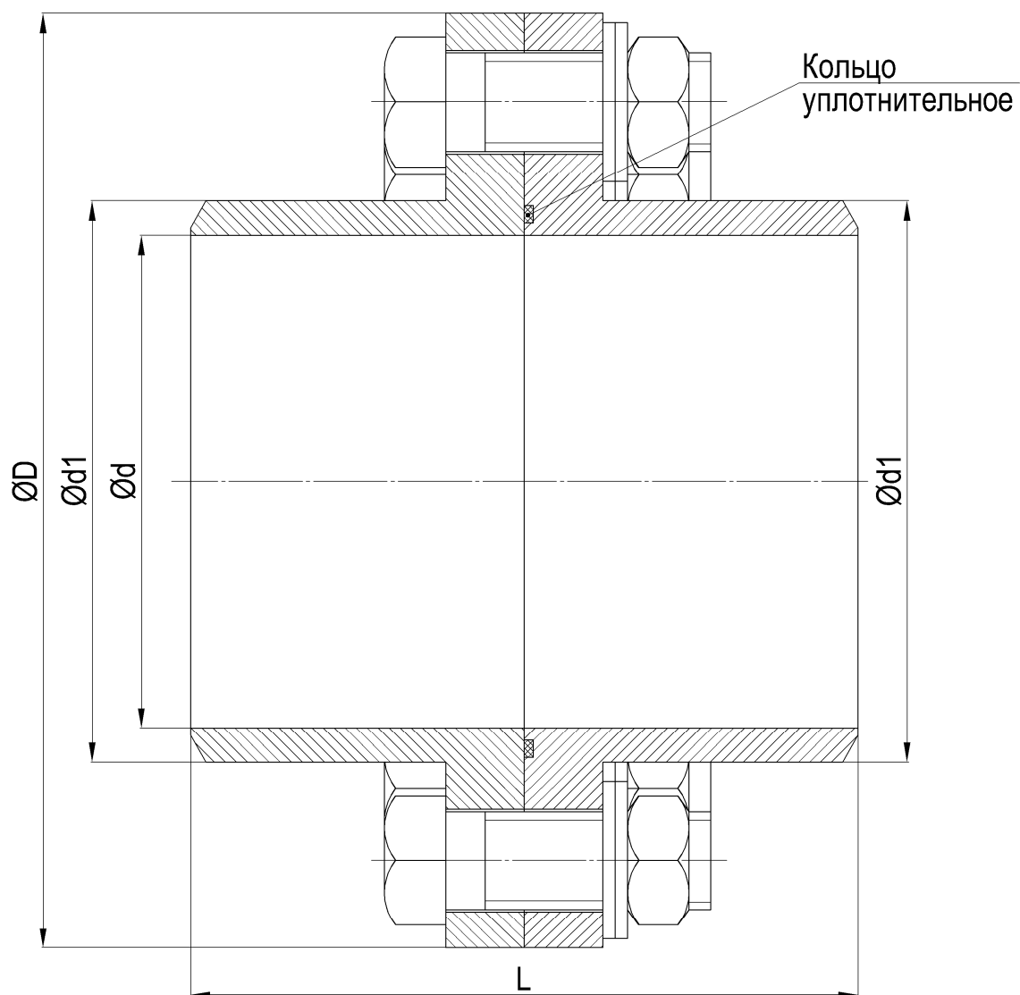
Рисунок 1 – Общий вид фланцевого соединения Ф
