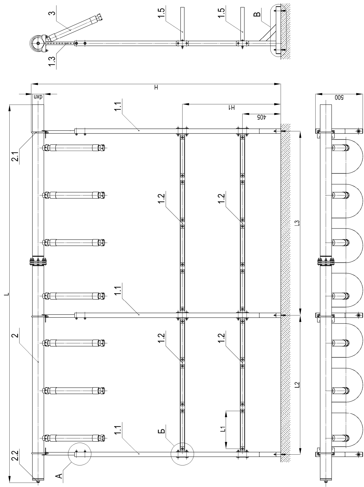
Рисунок А.2 – Общий вид стоек СМам-7...СМам-10 (остальное – см. рисунок А.1)
