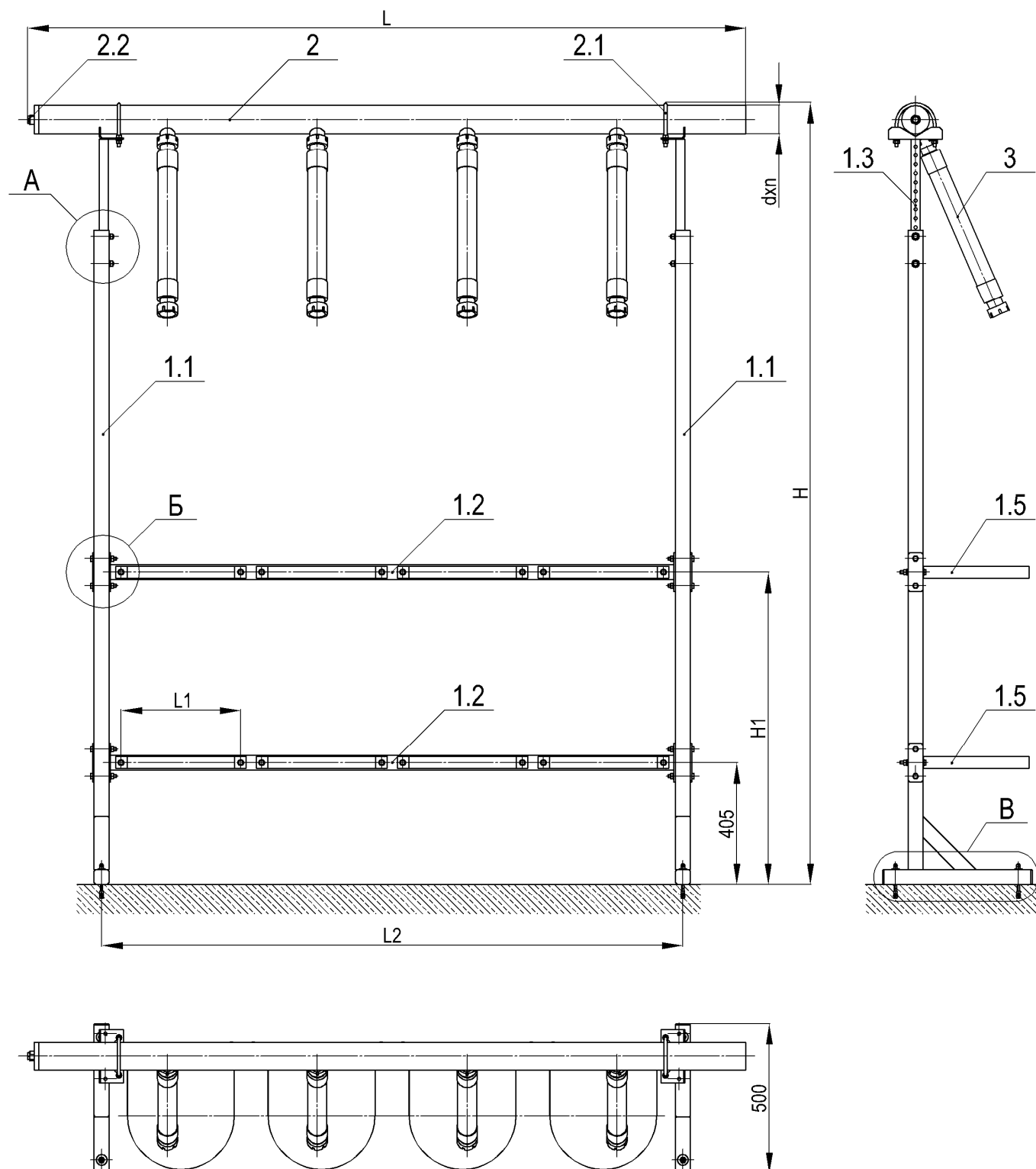
Рисунок А.1 – Общий вид стоек СМам-2...СМам-6 (лист 1 из 2)
