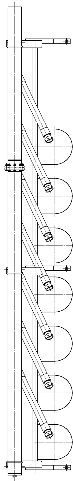
Рисунок А.2 – Общий вид стоек СМНм-7...СМНм-10 (остальное – см. рисунок А.1)
