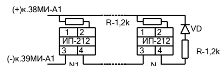
Шлейфы 1 помещений 1-3
