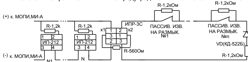
Схема шлейфов МОПИ и МИ-А с предупредительным сигналом "Внимание"
