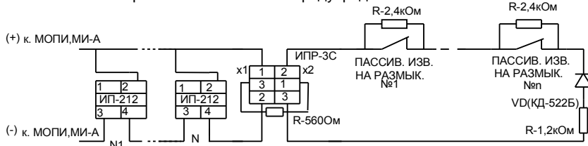
Схема шлейфов МОПИ и МИ-А без предупредительного сигнала "Внимание"
