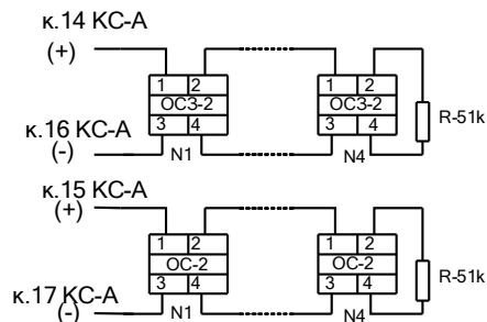
Шлейфы 2, 3, 4 помещений 1-2
