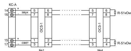
Схема подключения ОС3-1 (Пожар) на пожарном посту
