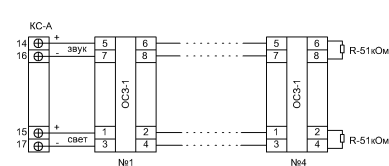
Схема подключения ОС3-1 (Пожар) на пожарном посту
