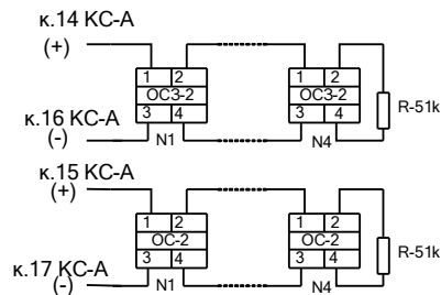
Схема подключения ОС32(Газ уходит), ОС-2(Газ не входит)
