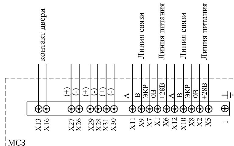
Рисунок 1 – Схема подключения модуля МСЗ.
